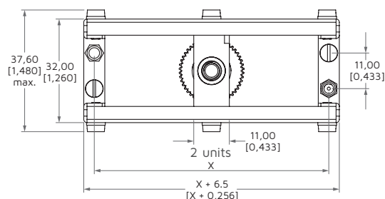
LEBVL Receptacle
