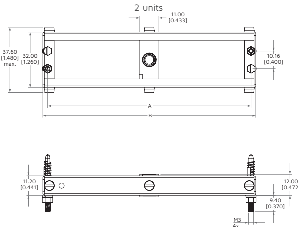
LEMVS Receptacle
