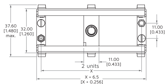
LEBVL Receptacle
